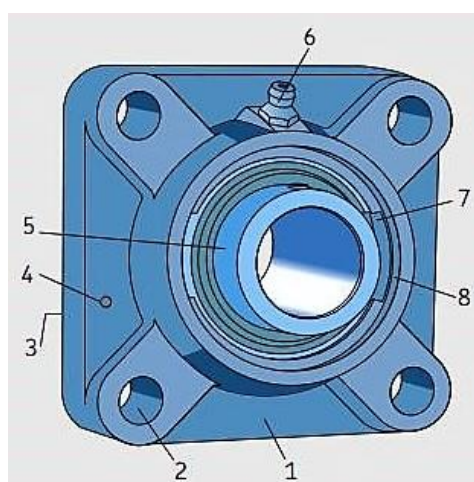
Slika 31. Jedinica Y-ležaja
