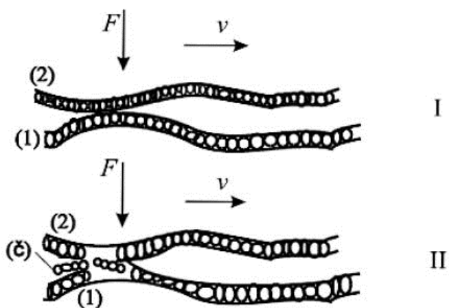
Slika 10. Jedinični događaj tribokorozije (Izvor: Grilec i sur., 2017.)
