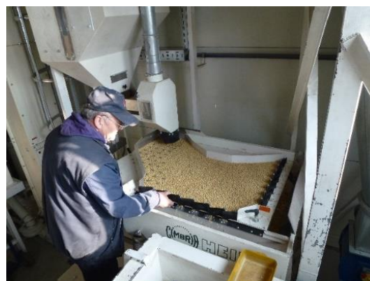
Slika 15. Gravitacijski stol (foto original; D. Galić Subašić)
