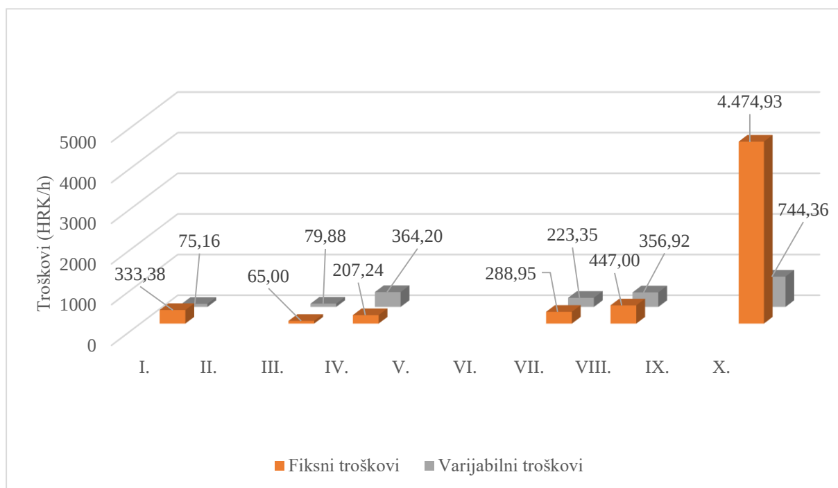
Grafikon 28. Fiksni i varijabilni troškovi rabljenih kombajna
