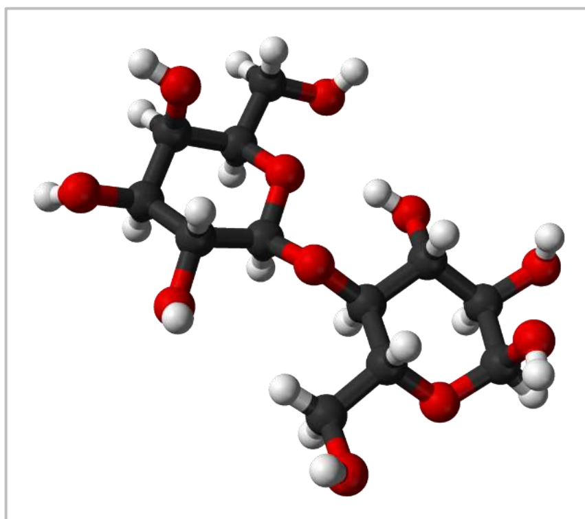
Slika 4. Molekula laktoze
