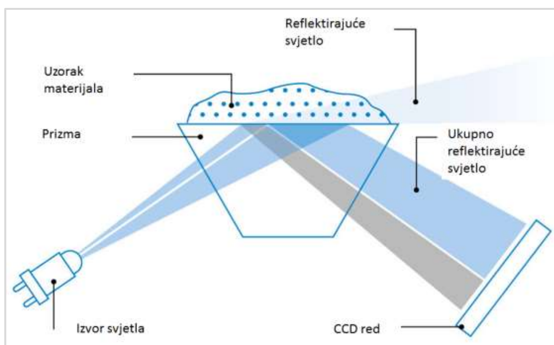
Slika 16. Princip refraktometrije
