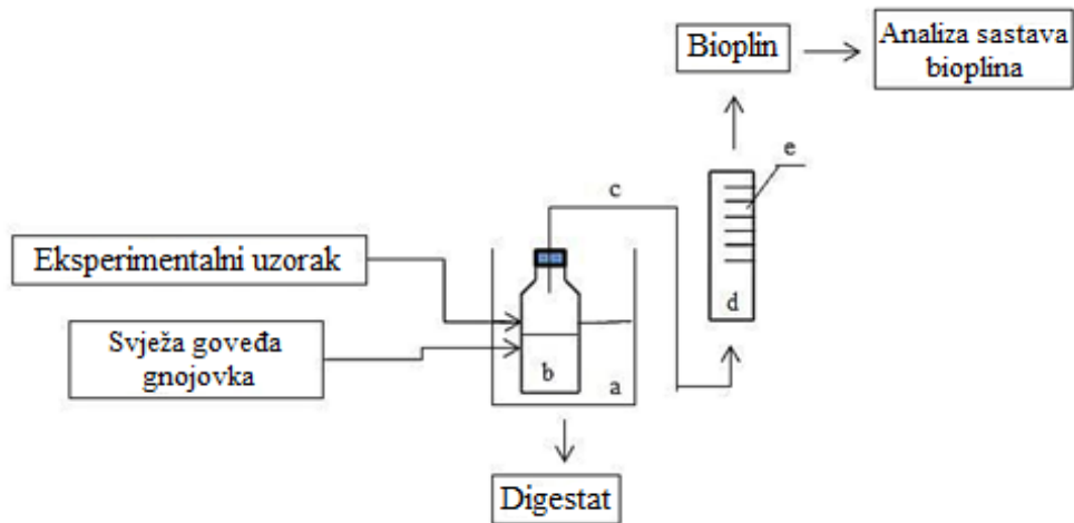
Slika 9. Shematski prikaz provedbe procesa anaerobne fermentacije
