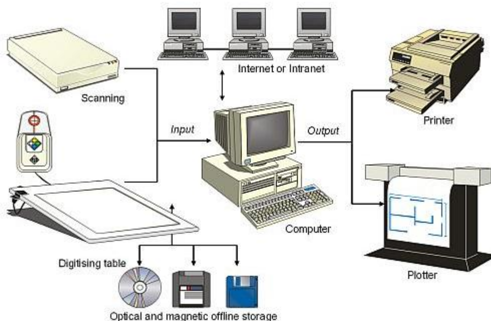
Slika 4. Hardware GIS-a
