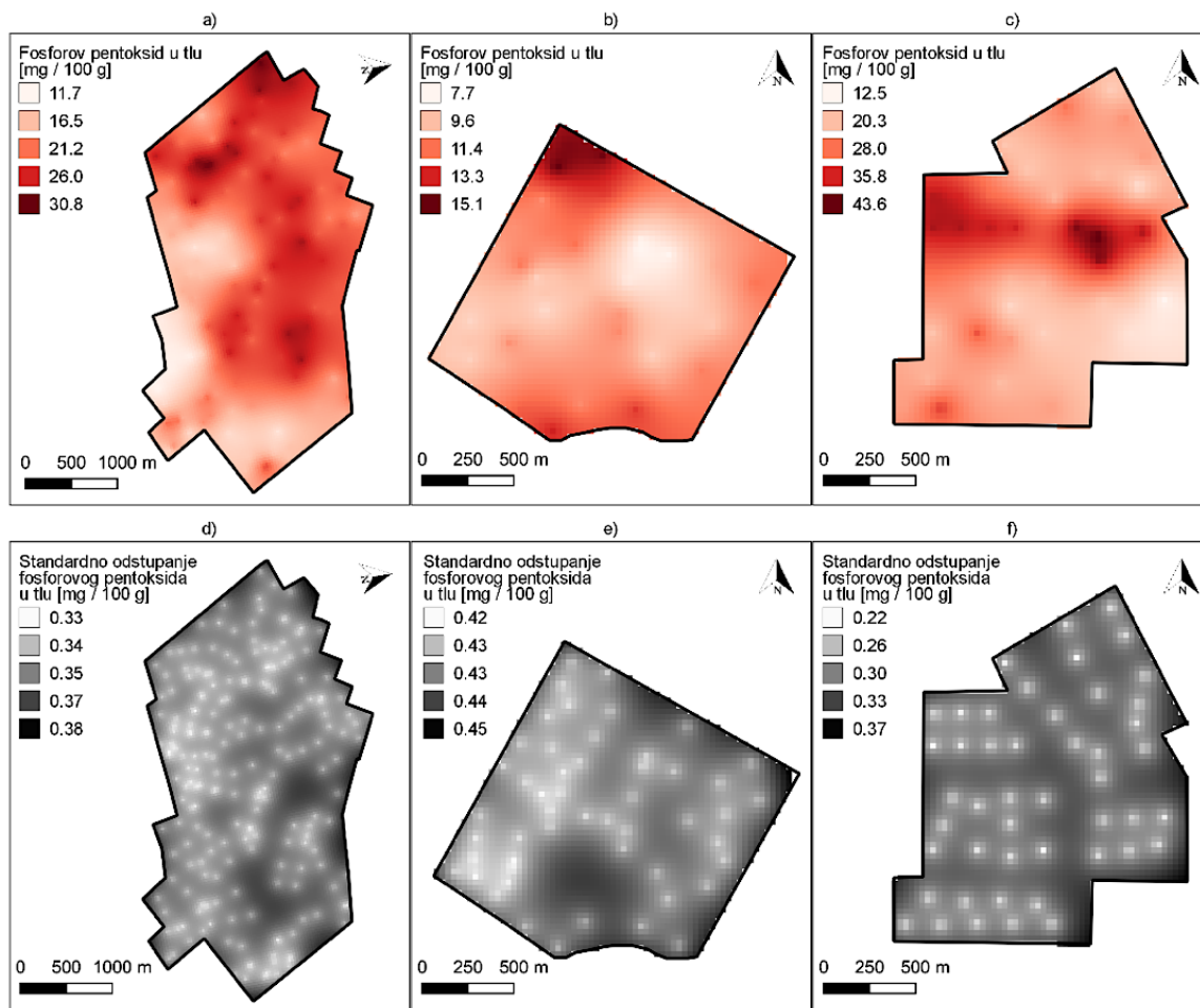
Slika 25. Sadržaj P 2 O 5 u tlu za: a) područje 1, b) područje 2, c) područje 3 te standardno odstupanje interpoliranih vrijednosti za: d) područje 1, e) područje 2, f) područje 3 (Izvor: Antonela Lončar, 2019.)
