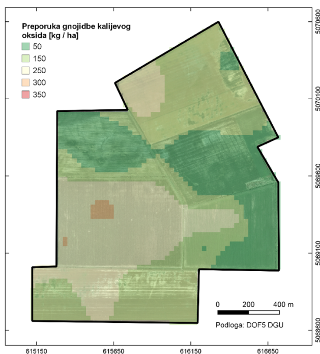
Slika 28. Preporuka gnojidbe kalijevog oksida
