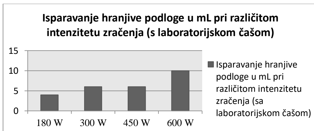
Grafikon 2. Isparavanje hranjive podloge u mL pri različitom intenzitetu zračenja (s laboratorijskom čašom), Izvor: Izrada autora
