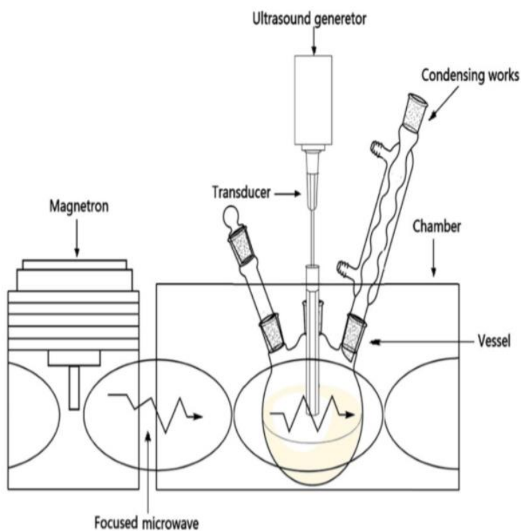
Slika 19: Shematski prikaz uređaja za ultrazvučno-mikrovalnom ekstrakciju (UMAE)
