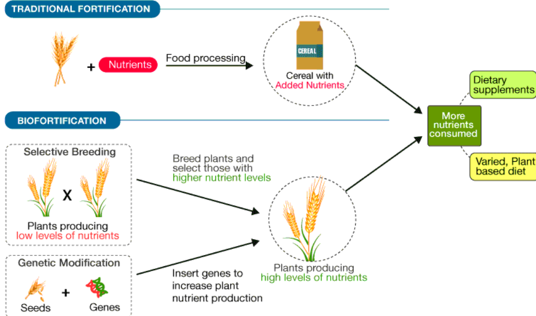
Slika 1. Shema biofortifikacije
