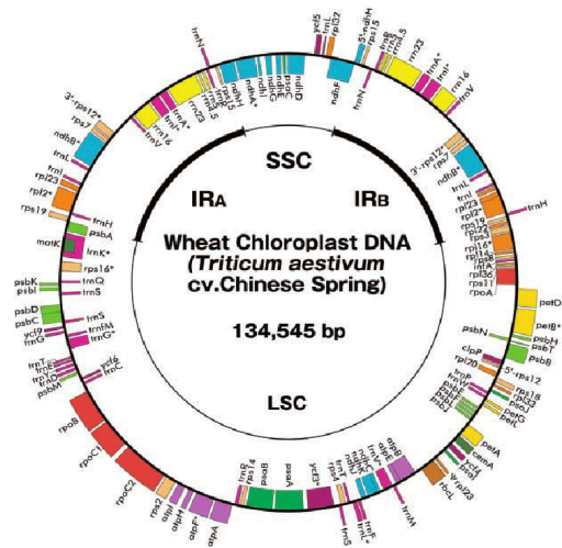
Slika 4. Kružna struktura genoma kloroplasta Triticum aestivum
