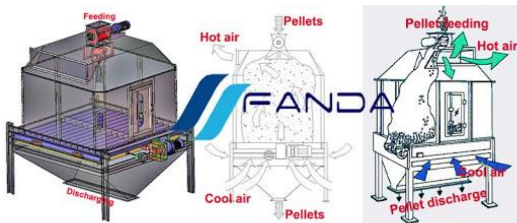
Slika 9. Vertikalni hladnjak
