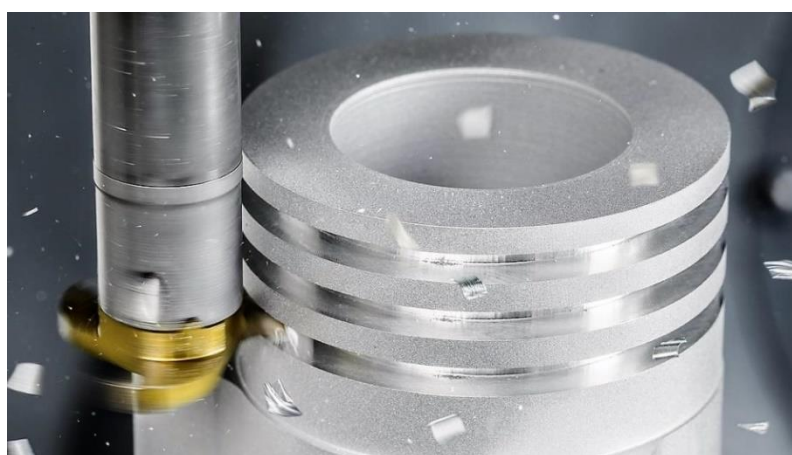
Slika 8. Glodanje aluminijskog klipa motora SUS ( https://www.nc-fertigung.de/besser-fraesen-in-aluminium )
