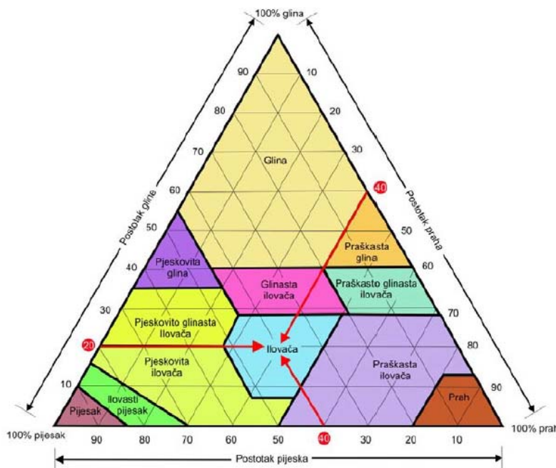
Slika 4. Atterbergov trokut za određivanje mehaničkog sastava tla. (Sofilić, 2014.)
