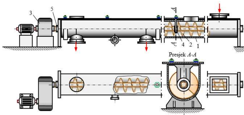
Slika 35. Sastav pužnog transportera s pogonskim mehanizmom (Izvor: Šumanovac i sur., 2011.)
