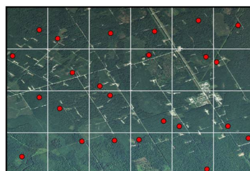
Stratificirano randomizirano uzorkovanje
