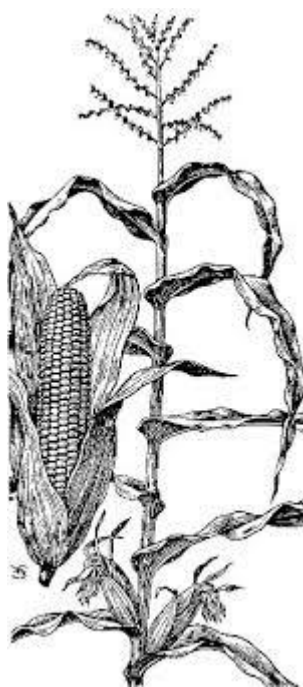
Slika 3. Stabljika kukuruza
