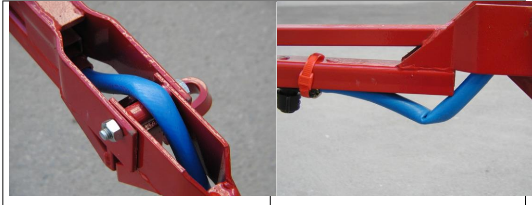
Slika 5. Nepravilno postavljene vodove tekućine (Izvor: Ivković I.)
