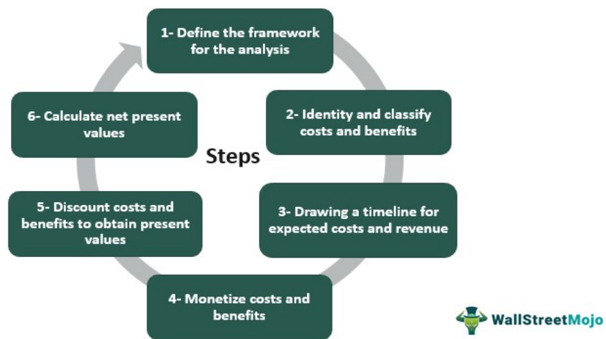
Slika 2. CBA analiza
