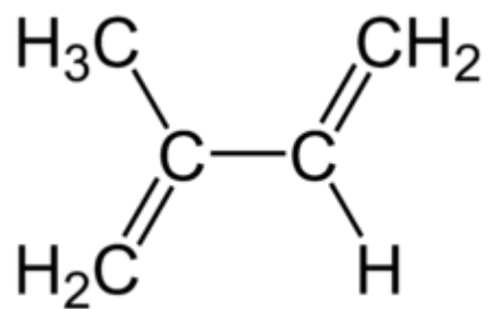
Slika 18. Izopren
