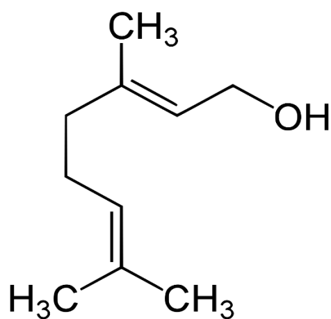
Slika 15. Geraniol
