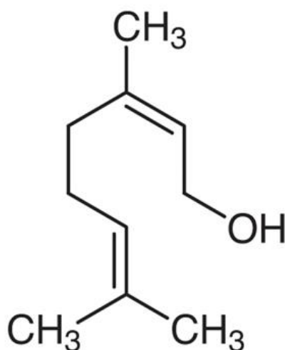
Slika 16. Nerol
