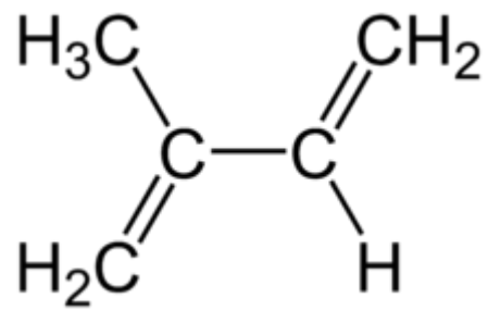
Slika 18. Izopren
