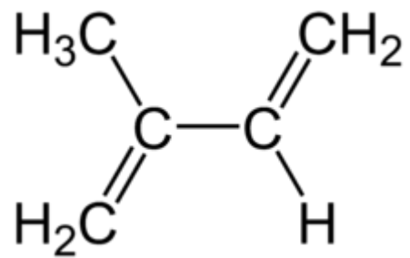
Slika 18. Izopren
