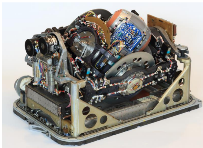
Slika 10. Kontrolni modul uređaja sa inercijskim navođenjem (Izvor: https://www.vectornav.com/resources/inertial-navigation-articles/what-is-an-ins )
