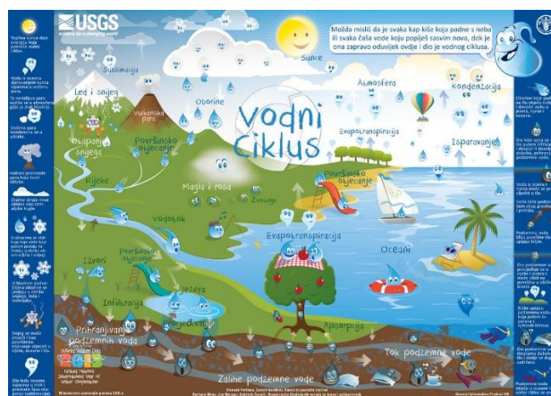
Slika 1. Hidrološki procesi
