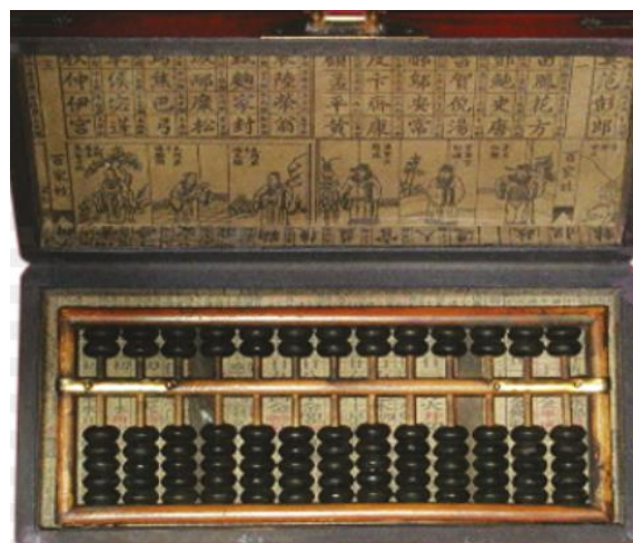
Slika 6. Abacus
