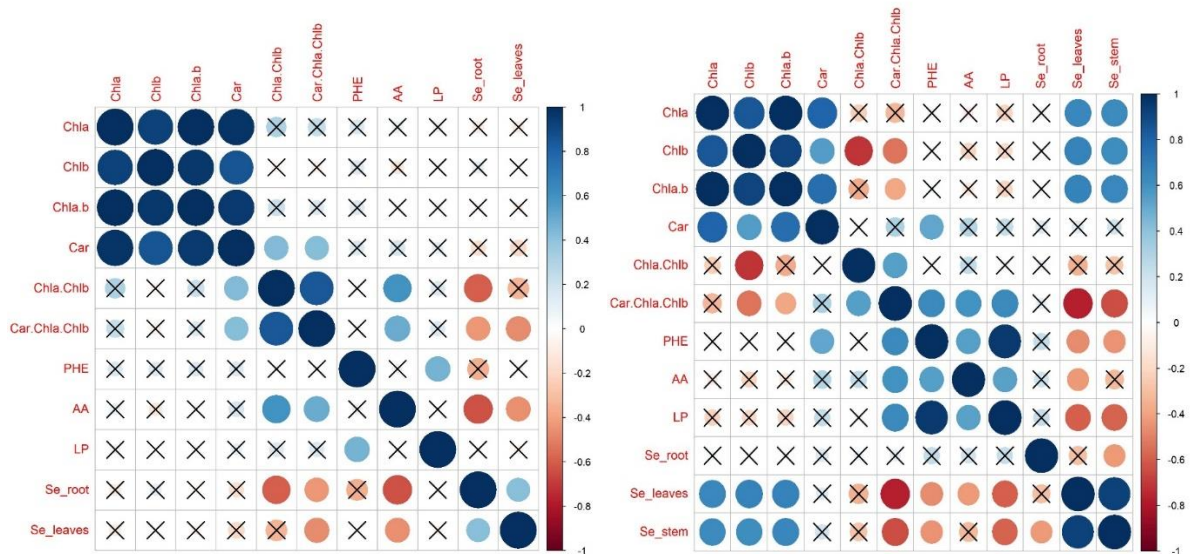
Slika 12. Korelacijski dijagrami (korelogram) prikazuju negativne (-, crvene) i pozitivne (+, plave) korelacije između fizioloških parametara i ukupnih koncentracija selena u listovima i korijenu matovilca (LIJEVO) i amaranta (DESNO). Izvor: Galić, neobjavljeni rezultati (2024.)
