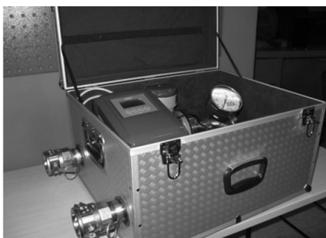
Slika 1. Elektromagnetni mjerjač kapaciteta crpke tvrtke Krohne
