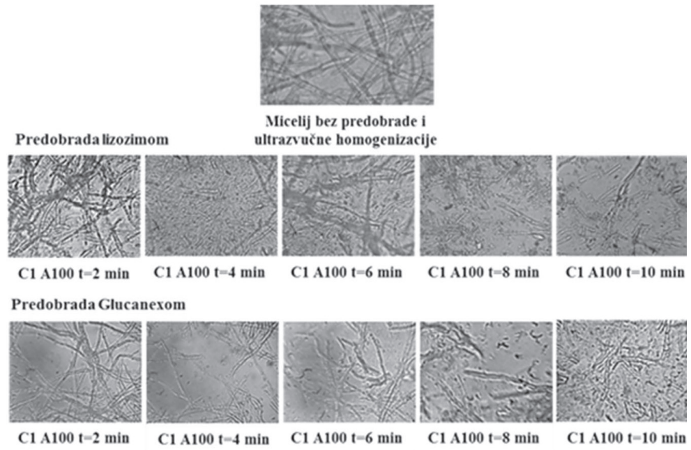
Slika 1. Mikroskopska analiza dezintegriranosti micelija. Prvi red: micelij prije predobrade i provođenja ultrazvučnog razbijanja. Drugi red: micelij nakon predobrade enzimskom razgradnjom lizozimom i provođenja ultrazvučnog razbijanja u vremenu od 2 do 10 minuta. Treći red: micelij nakon predobrade enzimskom razgradnjom Glucanex -om i provođenja ultrazvučnog razbijanja u vremenu od 2 do 10 minuta.
