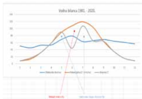
Grafikon 4b. Vodna bilanca prema Thornthwaiteu na području Orahovice (RH) za razdoblje 1981. – 2020. godine
