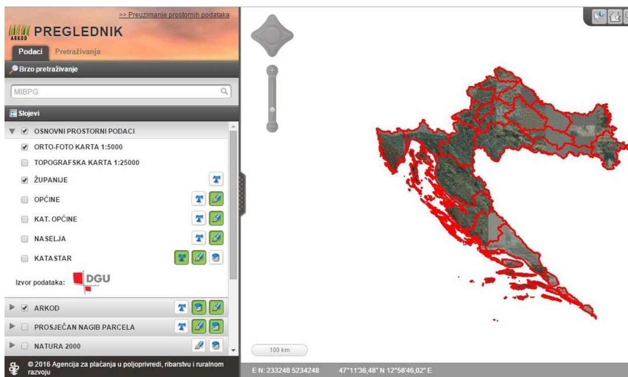
Slika 3. ARKOD preglednik
