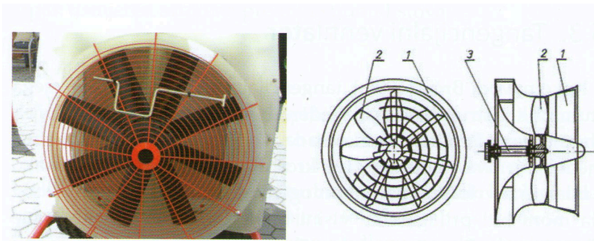
Slika 13. Aksijalni ventilator (1-kućište, 2-lopatice, 3-vratilo ventilatora)
